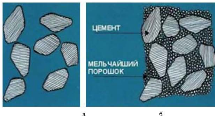
Рис. 2. Структура бетона: а – без содержания микрокремнезема, б – с содержанием микрокремнезема.
