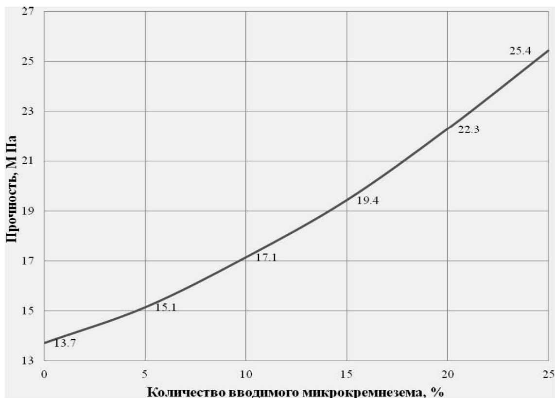
Рис. 1. Зависимость прочности бетона от содержания микрокремнезема..
