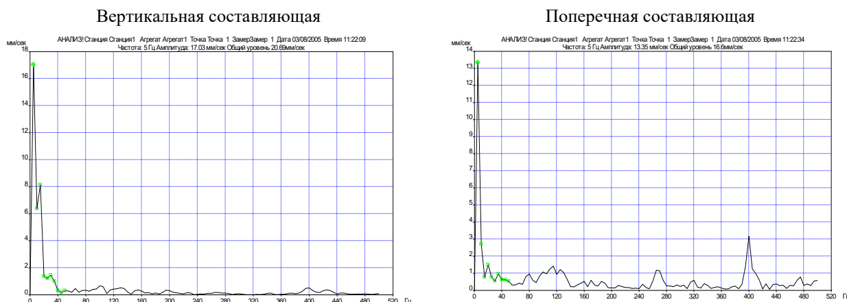
Рис. 5. Интенсивность вибрации на редукторе ленточного перегружателя Fig. 5. Intensity of vibration on the gearbox belt loader
