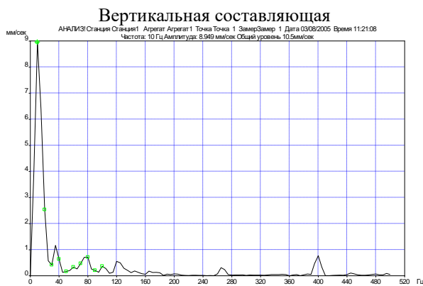
Рис. 4. Интенсивность вибрации на заднем подшипнике гидродвигателя ленточного перегружателя
