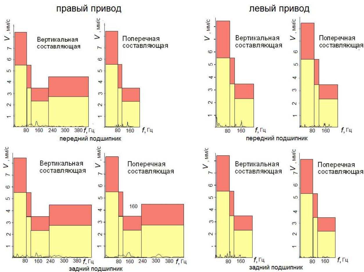
Рис. 2. Обобщенные спектральные маски для приводов режущей части комплекса Superior Highwall Miners Fig. 2. Generalized spectral masks for drives of the cutting part of the Superior Highwall Miners complex
