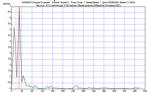
Рис. 6. Интенсивность вибрации на двигателе скребкового конвейера Fig. 6. Intensity of vibration on the scraper conveyor motor
