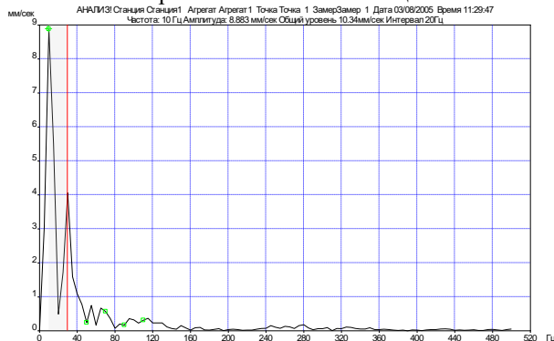
Рис. 6. Интенсивность вибрации на двигателе скребкового конвейера Fig. 6. Intensity of vibration on the scraper conveyor motor
