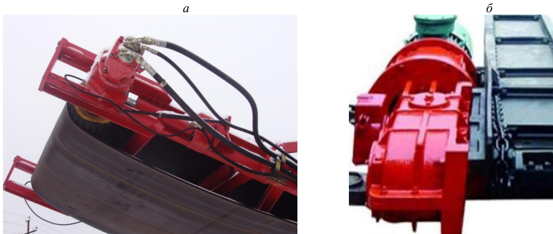
Рис. 3. Привода скребкового конвейера (а) и ленточного перегружателя (б) комплекса Superior Highwall Miners
