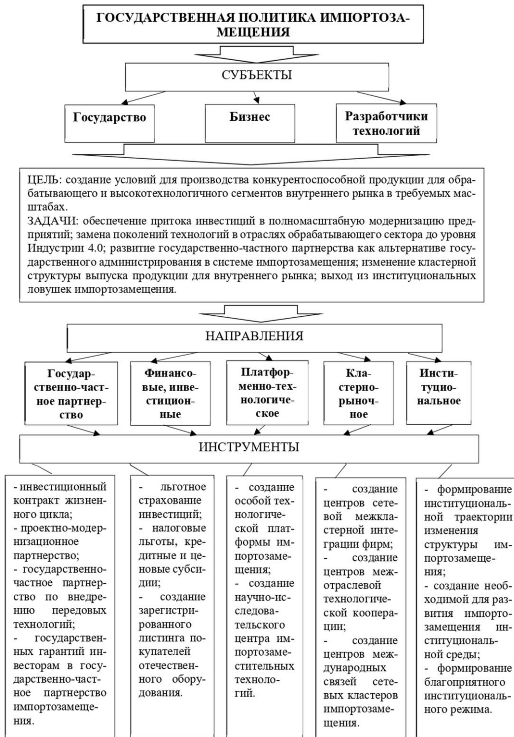
Рис. 1. Схема формирования и реализации государственной политики импортозамещения (составлен авторами)
